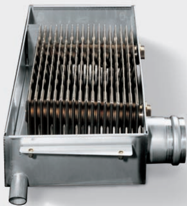
Das Edelstahlgliederprofil des Kondensationswärmetauschers sorgt für eine optimale Energieausnutzung
